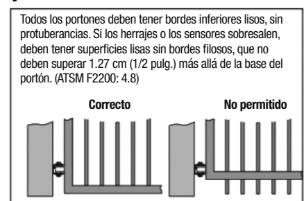
Base del portón pivotante y deslizando FIGURA 5
