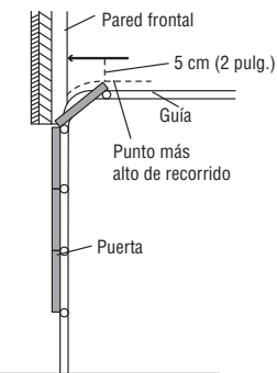
Puerta seccional con guía curva
