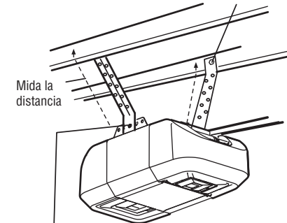
Perno hexagonal de 5/16 de pulg.-18 x 7/8 de pulg., Arandela de presión de 5/16 de pulg., Tuerca de 5/16 de pulg.-18
