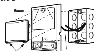
Figura 2 INSTALACIÓN PRECABLEADA
